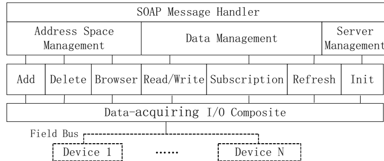
Fig. 3. Configuration of OPC XML-DA module
